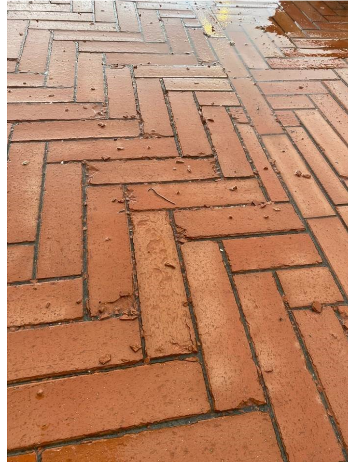
Mattonelle posate meno di un anno fa in stato di degradazione Febbraio 2020
